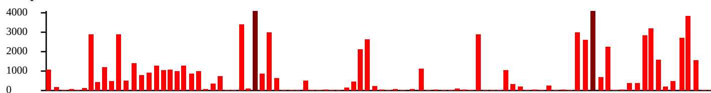
siliqueLate_0
